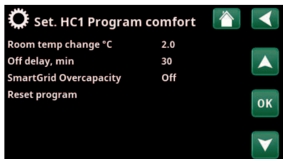
Menu: „Zaawansowany\Ustawienia\Obieg grzewczy\Obieg grzewczy 1/Program/Komfort”.
