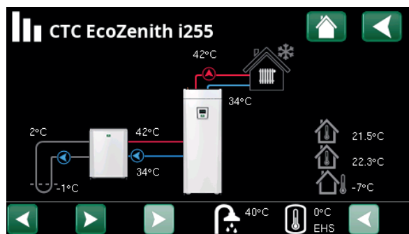
Wyświetlacz pokazuje informacje o pracy z podłączoną pompą ciepła CTC EcoPart.
